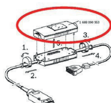
Moduł U-BOX2 do KTS 520/550/650
