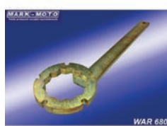
Klucz M60 / 12 kątny do blokowania koła pasowego wałka rozrządu Subaru
